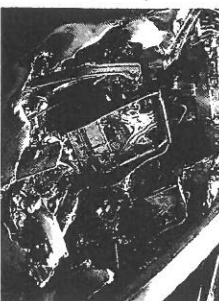
Abb. 3: LKA Berlin. BMW-Cabrio, massive Brandzerstörung, auf dem Fahrsitz teilweise brannter Papierspiel.
